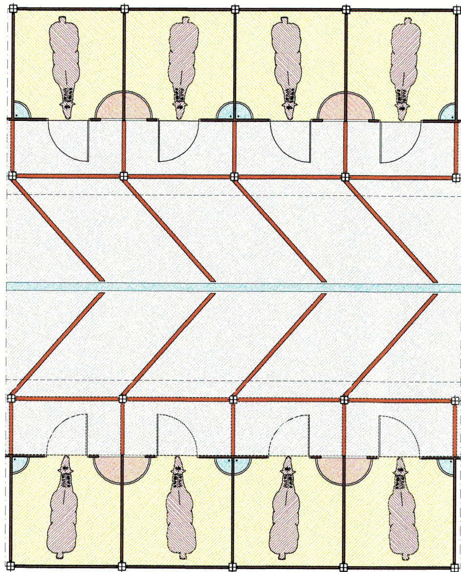
PLANTA DE CUADRAS
